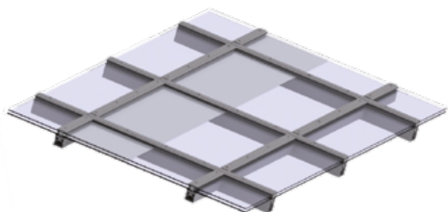
Système d'ombrage intégré au vitrage
